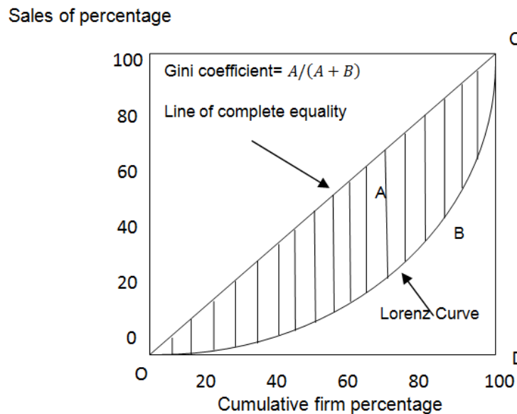
Fig. 2. Lorenz Curve
